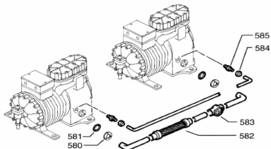
550 - Комплект для разгрузки пуска
