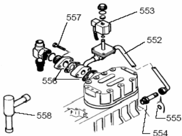
Линия уравнивания по маслу для 2 компрессоров
