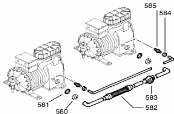
580 - Линия уравнивания по маслу для 2 компрессоров
