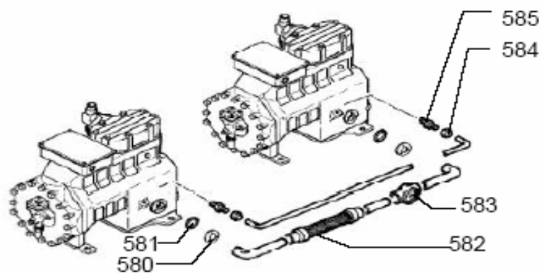
Линия уравнивания по маслу для 2 компрессоров
