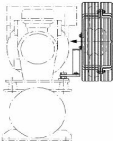
550- Комплект для разгрузки пуска
