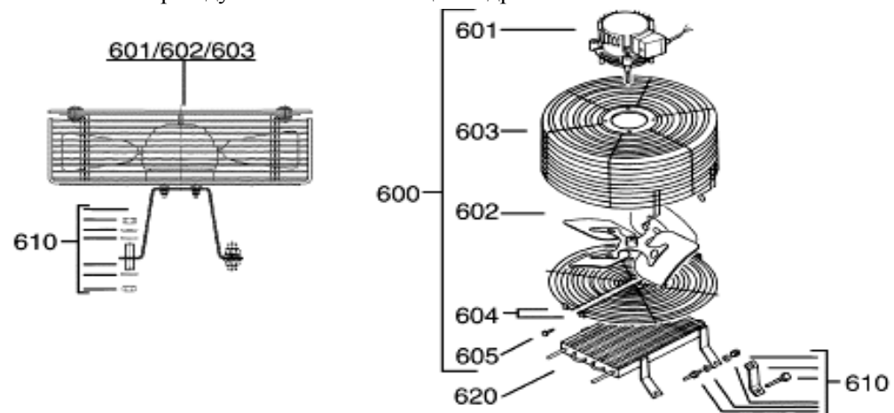
600 - Вентилятор обдува головки блока цилиндров
