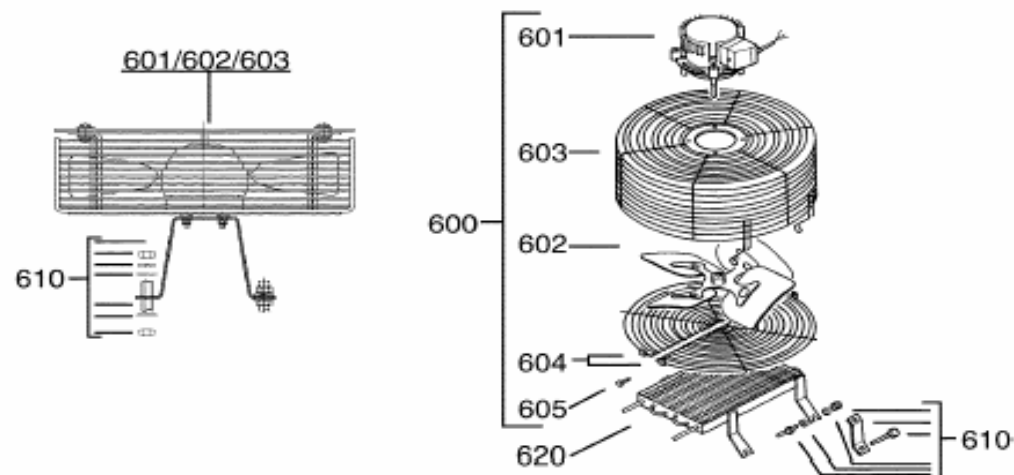
600- Вентилятор обдува головки блока цилиндров
